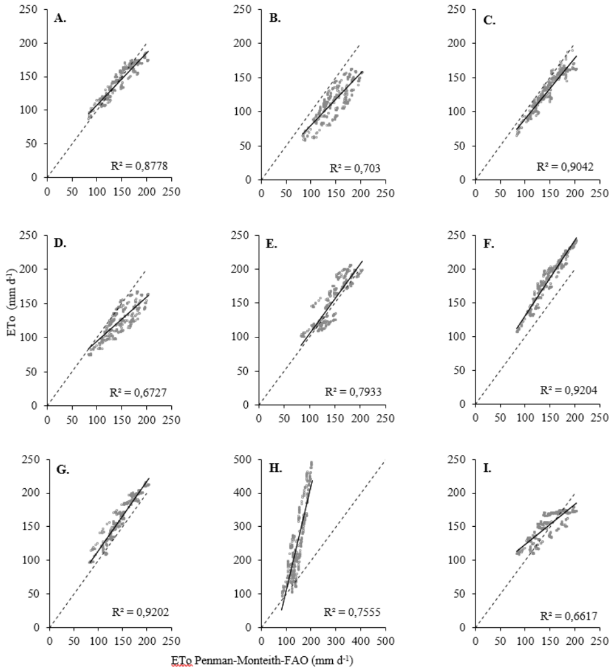
Figura 2. Comparação da evapotranspiração de referência média mensal (1995-2014) em mm mês -1 entre o método Penman-Monteith-FAO e os métodos avaliados, evidenciando a reta gerada por meio de regressão linear e a linha tracejada 1:1. Métodos avaliados: Hargreaves-Samani (A); Thornthwaite-48 (B); Thornthwaite modificado por Camargo (C); Camargo-71(D); Blaney-Criddle (E); Jensen-Haise (F); Radiação FAO-24 (G); Aerodinâmico (H) e Energético (I).
