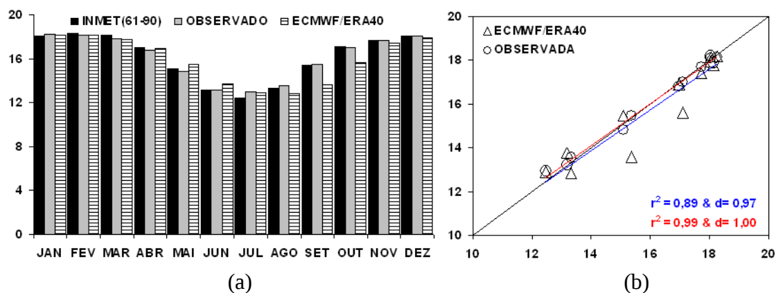
Figura 8 – Climatologia da temperatura mínima, °C, da mesorregião Jequitinhonha (MR04), no período de 1961 a 1990 – PRESENTE (a); validações das séries de dados observados e do ECMWF/ERA40 (na abscissa climatologia oficial do INMET) (b).
