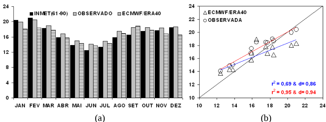
Figura 10 – Climatologia da radiação global incidente, em MJ/m 2 d, da mesorregião Jequitinhonha (MR04), no período de 1961 a 1990 – PRESENTE (a); validações das séries de dados observados e do ECMWF/ERA40 (na abscissa climatologia oficial do INMET) (b).
