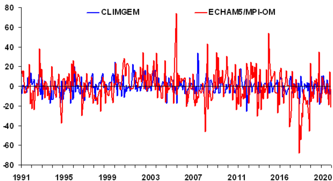
Figura 21E – Anomalias mensais de evapotranspiração de referência estimada com registros meteorológicos simulados pelo CLINGEN (séries sintéticas) e ECHAM5/MPI-OM (série dinâmica) para Mesorregião Central Mineira (MR09), em mm/mês, no período de 1991 a 2020 – FUTURO.
