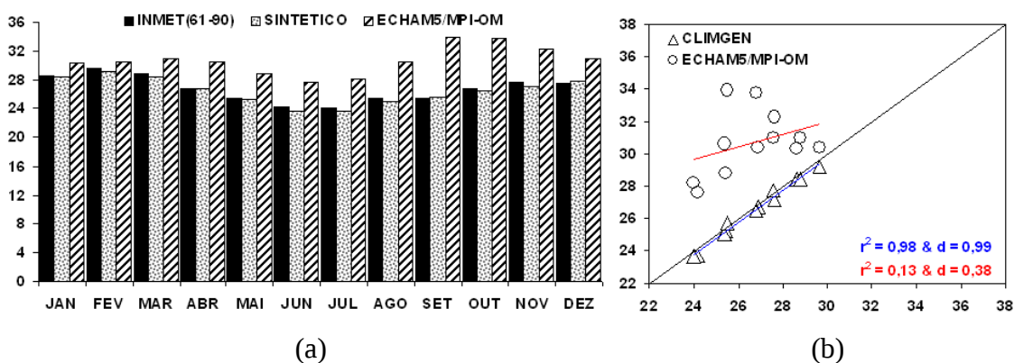
Figura 5H – Climatologia da temperatura máxima, em °C, da Mesorregião Zona da Mata Mineira (MR12), no período de 1991 a 2020 – FUTURO (a); validações entre as climatologias das séries simuladas pelo CLIMGEN e o ECHAM5/MPI-OM (na abscissa climatologia oficial do INMET) (b).
