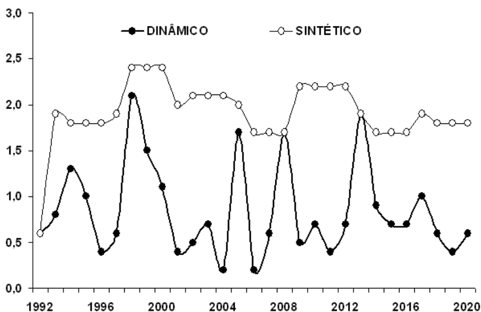
Figura 49 – Índice de área foliar máximo do cultivar BR201. Impactos e projeções do clima por meio de séries meteorológicas dinâmicas (ECHAM5/MPI-OM) e sintéticas (CLIMGEN) para Mesorregião Jequitinhonha (MR04).
