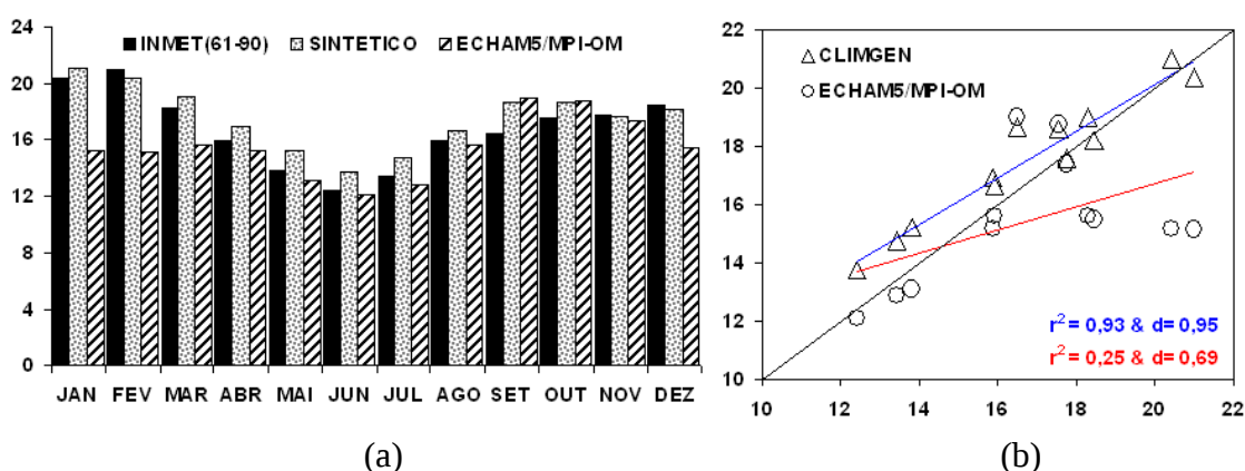
Figura 11 – Climatologia da radiação global incidente, em MJ/m 2 d, da mesorregião Jequitinhonha (MR04), no período de 1991 a 2020 – FUTURO (a); validações entre as climatologias das séries simuladas pelo CLIMGEN e o ECHAM5/MPI-OM (na abscissa climatologia oficial do INMET) (b).
