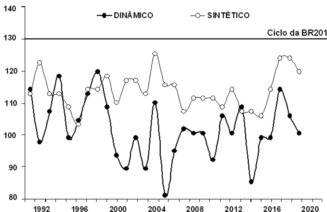
Figura 43 – Ciclo total do cultivar BR201, em dias. Impactos e projeções do clima por meio de séries meteorológicas dinâmicas (ECHAM5/MPI-OM) e sintéticas (CLIMGEN) para Mesorregião Jequitinhonha (MR04).
