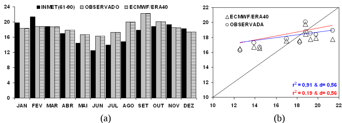
Figura 8E – Climatologia da radiação global incidente, em MJ/m²d, da mesorregião Central Mineira (MR09), no período de 1961 a 1990 – PRESENTE (a); validações das séries de dados observados e do ECMWF/ERA40 (na abscissa climatologia oficial do INMET) (b).
