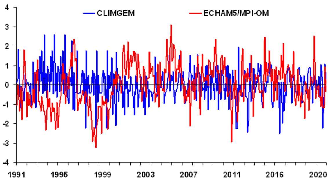
Figura 16G – Anomalias mensais de temperatura mínima dos registros simulados pelo CLIMGEN (séries sintéticas) e ECHAM5/MPI-OM (série dinâmica) para Mesorregião Triângulo Mineiro/Alto Paranaíba (MR11), em °C, no período de 1991 a 2020 – FUTURO.
