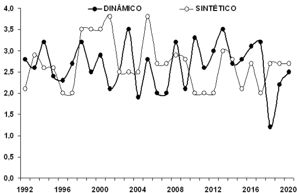
Figura 50 – Índice de área foliar máximo do cultivar BR201. Impactos e projeções do clima por meio de séries meteorológicas dinâmicas (ECHAM5/MPI-OM) e sintéticas (CLIMGEN) para mesorregião do Triângulo Mineiro e Alto Paranaíba (MR11).
