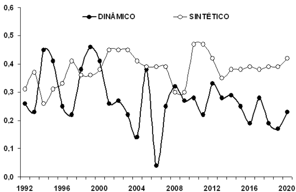
Figura 51 – Índice de colheita do cultivar BR201. Impactos e projeções do clima por meio de séries meteorológicas dinâmicas (ECHAM5/MPI-OM) e sintéticas (CLIMGEN) para Mesorregião Jequitinhonha (MR04).
