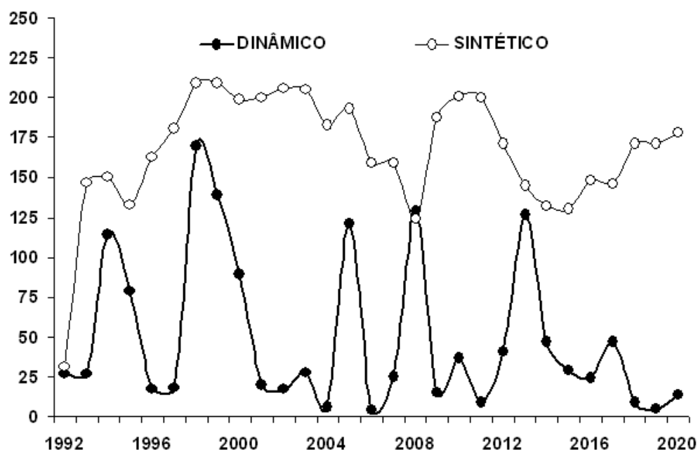
Figura 47 – Transpiração total, em mm. Ciclo total do cultivar BR201, em dias. Impactos e projeções do clima por meio de séries meteorológicas dinâmicas (ECHAM5/MPI-OM) e sintéticas (CLIMGEN) para Mesorregião Jequitinhonha (MR04).
