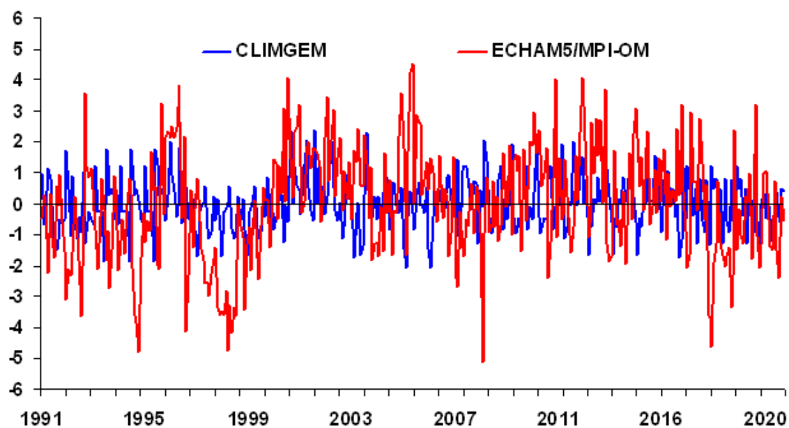
Figura 15B – Anomalias mensais de temperatura máxima a partir de “registros simulados pelo CLIMGEM (séries sintéticas) e ECHAM5/MPI-OM (série dinâmica)” para mesorregião Sul e Sudoeste de Minas (MR01), em °C, no período de 1991 a 2020 – FUTURO.
