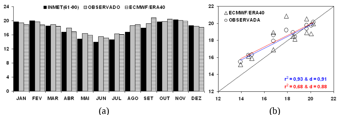
Figura 7G – Climatologia da radiação global incidente, em MJ/m²d, da Mesorregião Triângulo Mineiro/Alto Paranaíba (MR11), no período de 1961 a 1990 – PRESENTE (a); validações das séries de dados observados e do ECMWF/ERA40 (na abscissa climatologia oficial do INMET) (b).
