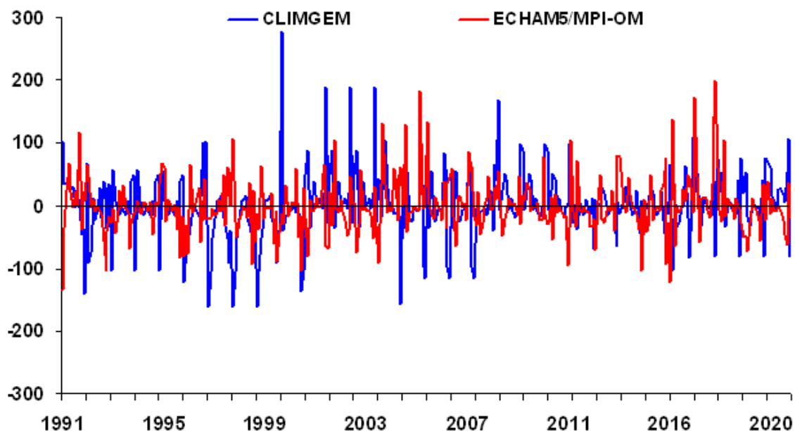
Figura 13F – Anomalias mensais de precipitação total dos “registros simulados pelo CLIMGEM (séries sintéticas) e o ECHAM5/MPI-OM (série dinâmica)” para Mesorregião de Belo Horizonte (MR10), em mm/mês, no período de 1991 a 2020 – FUTURO.
