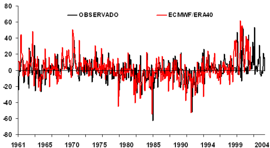
Figura 19G – Anomalias mensais de evapotranspiração de referência dos registros observado e reanálise do ECMWF/ERA40 para Mesorregião Triângulo Mineiro/A. Paranaíba (MR11), em mm/mês. Período 1961 a 2002 para ECMWF/ERA40 e 1961 a 2004 para o observado – PRESENTE.
