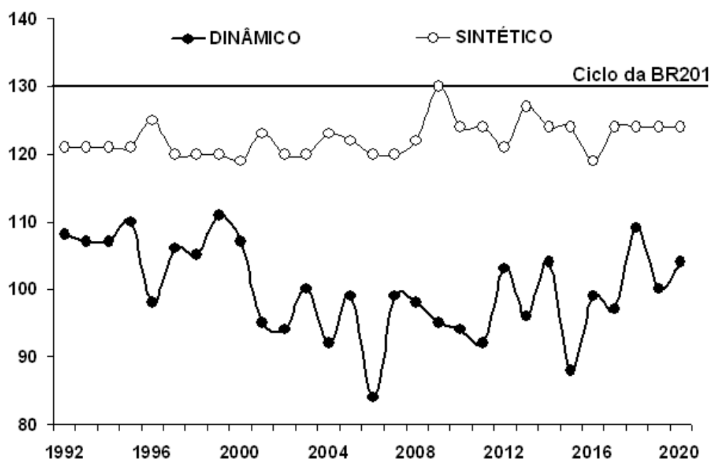
Figura 44 – Ciclo total do cultivar BR201, em dias. Impactos e projeções do clima por meio de séries meteorológicas dinâmicas (ECHAM5/MPI-OM) e sintéticas (CLIMGEN) para mesorregião do Triângulo Mineiro e Alto Paranaíba (MR11).
